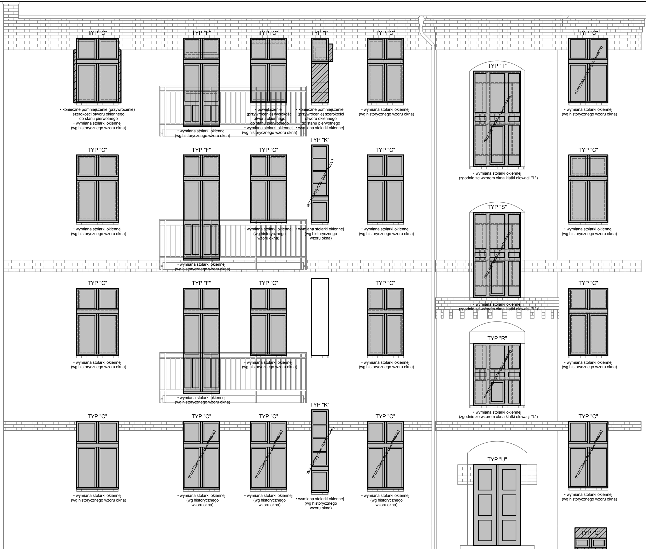
ELEWACJA "D"
