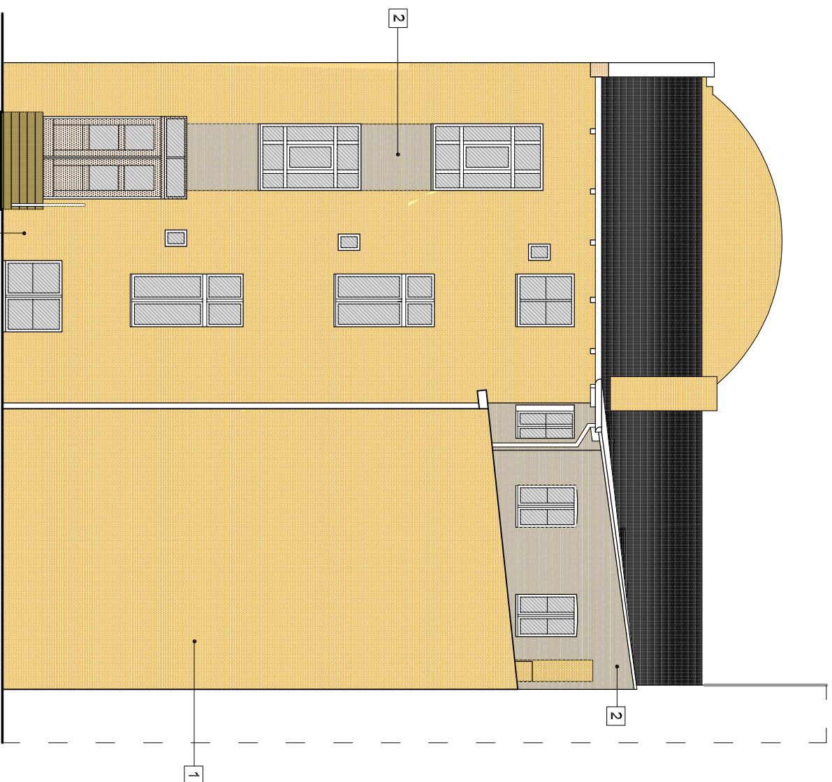
ELEWACJA POŁUDNIOWO - WSCHODNIA
