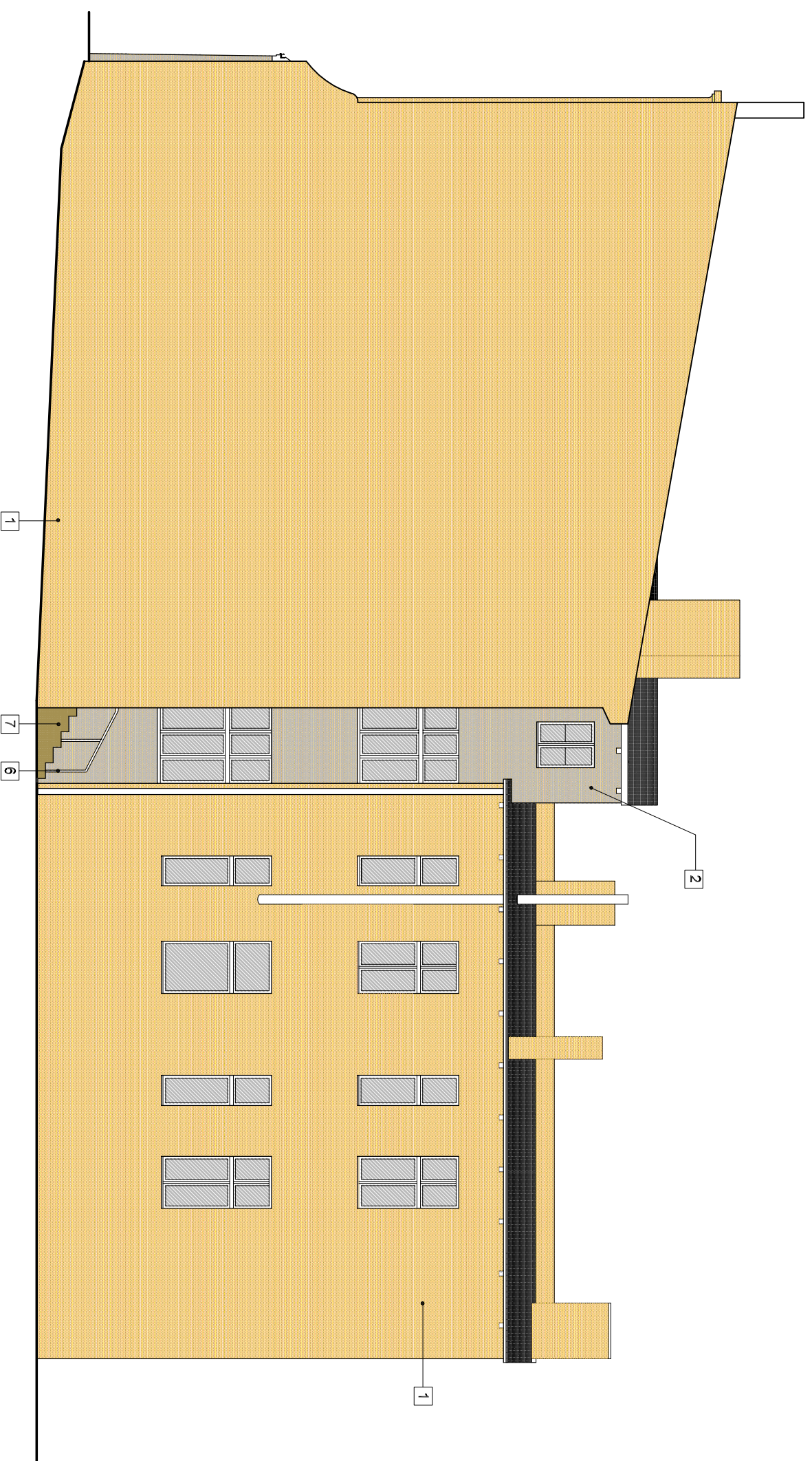
ELEWACJA POŁUDNIOWO - ZACH.
