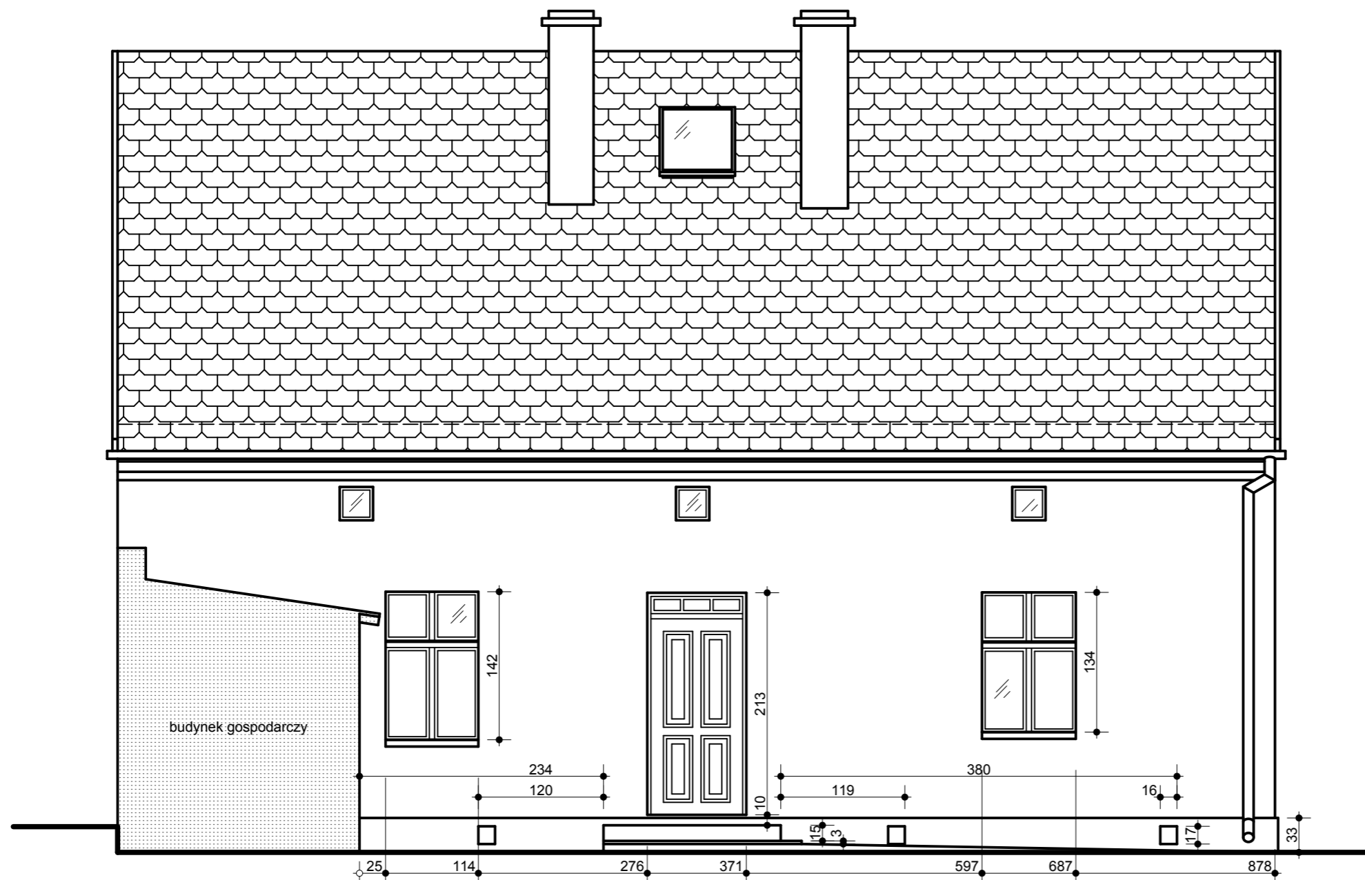
ELEWACJA POŁUDNIOWA "E" (PODWÓRKOWA)
