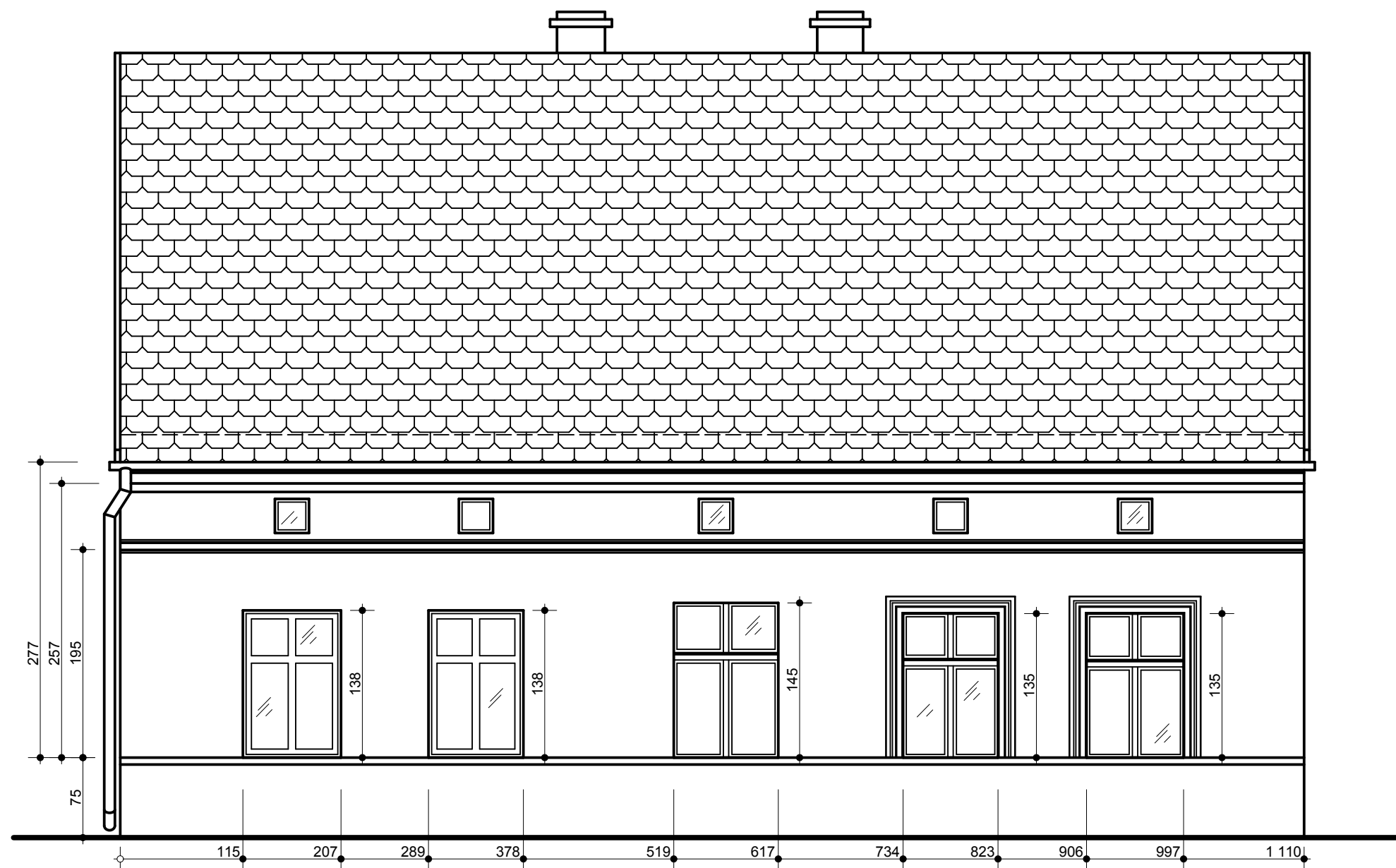
ELEWACJA PÓŁNOCNA "A" (FRONTOWA)
