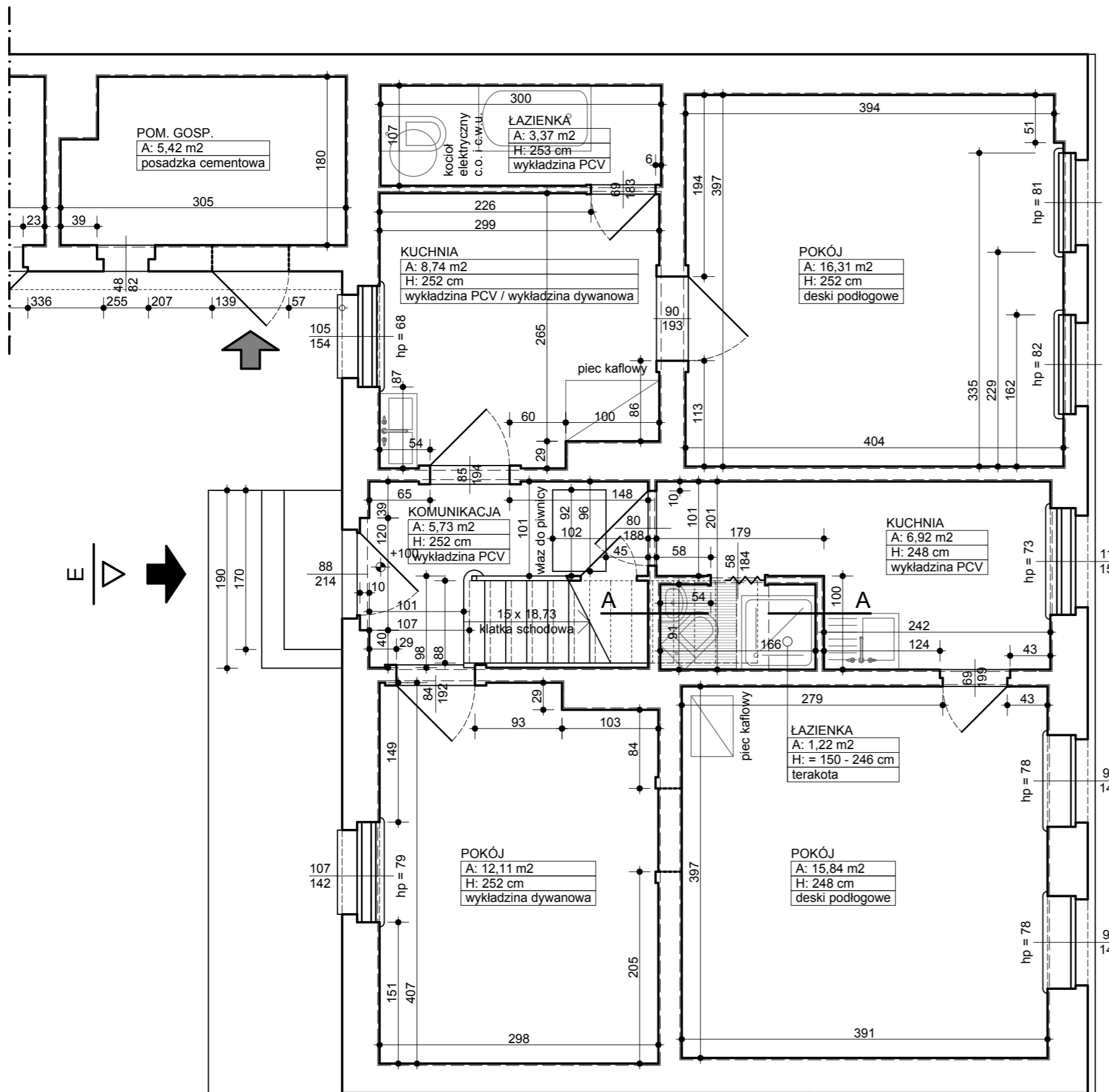
BUDYNEK MIESZKALNY: RZUT PARTERU
