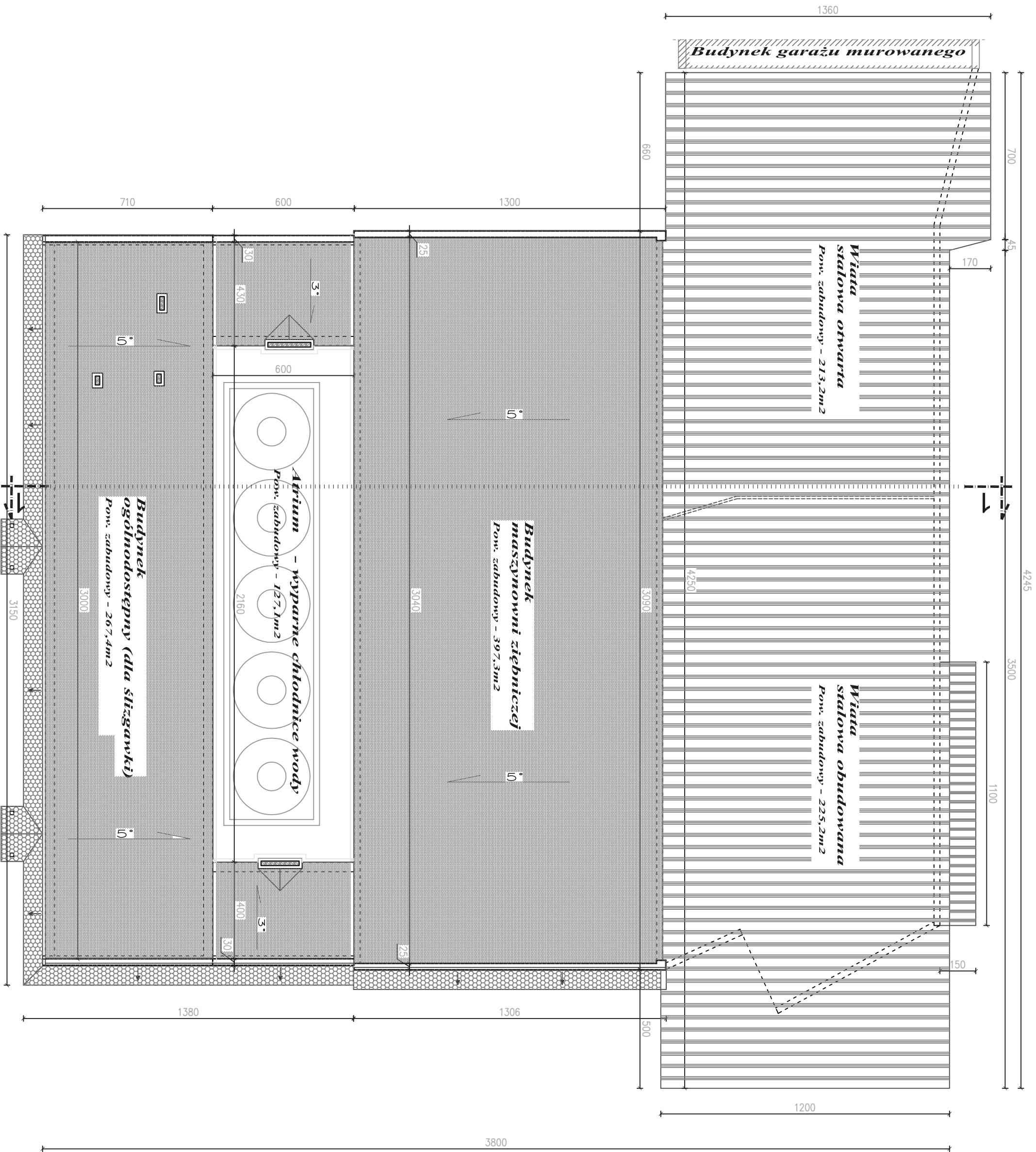
RZUT DACHU SKALA 1:150
