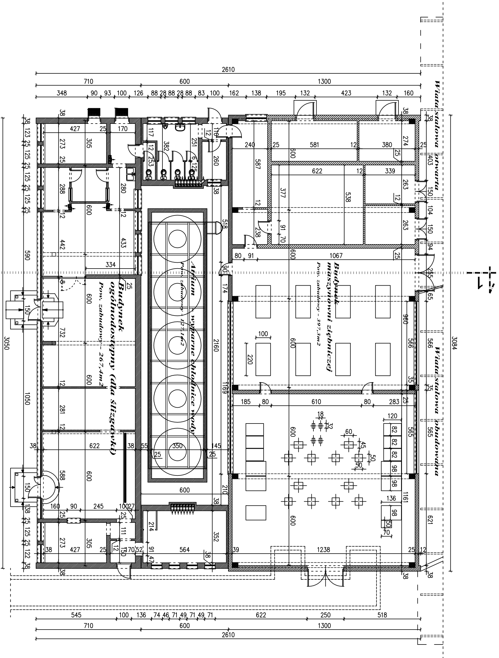
RZUT PRYZIEMIA SKALA 1:150
