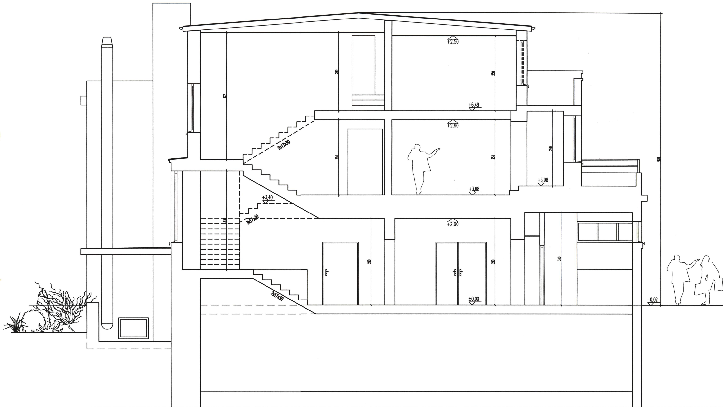
PRZEKRÓJ A/A
