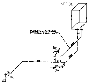
AKSONOMETRIA 1:50
