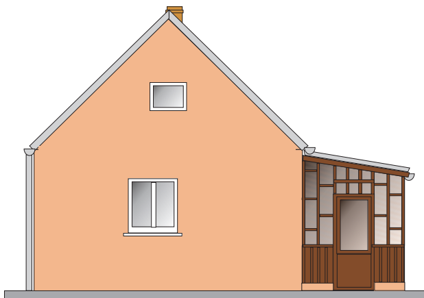
Ściana szczytowa
