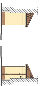
PORTALE nr 2, 3 i 4 bok lewy
