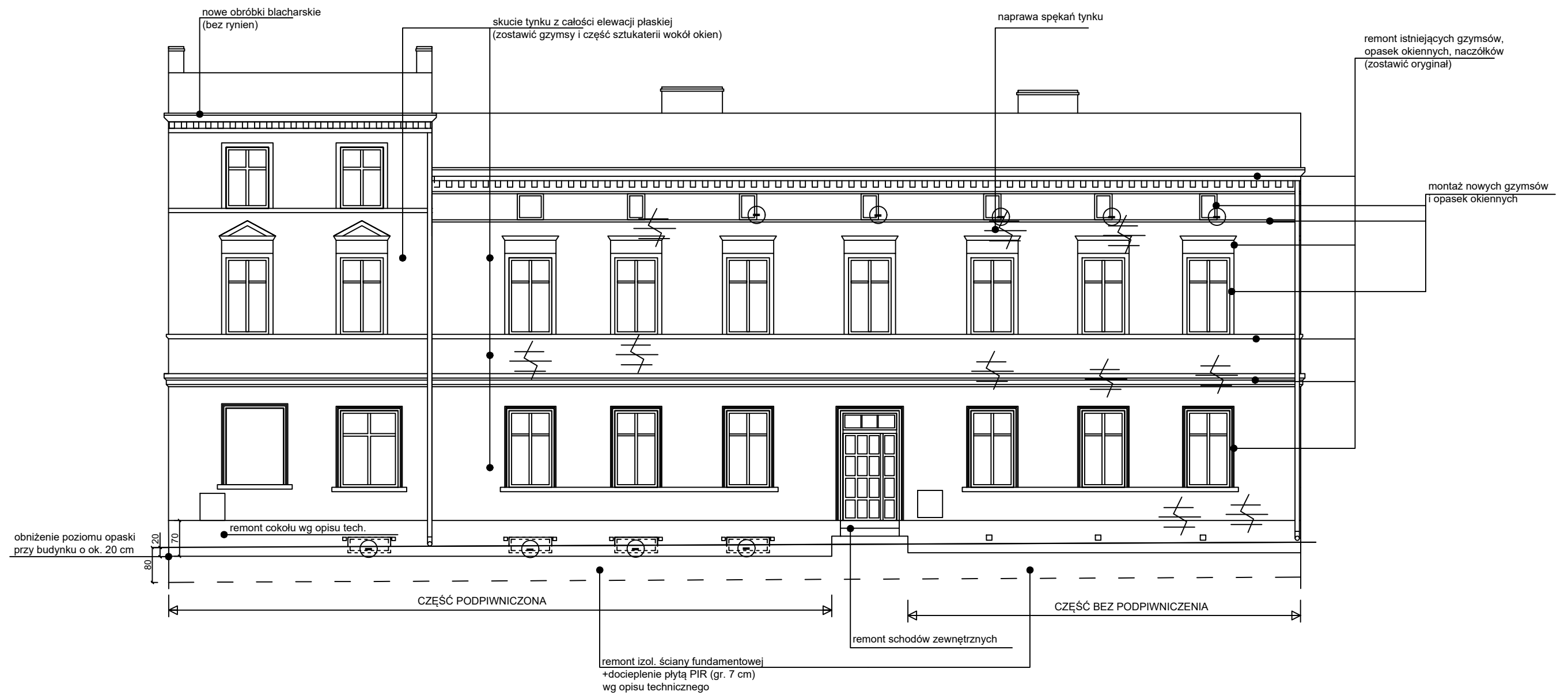
ELEWACJA PÓLNOĆNA SKALA 1:100
