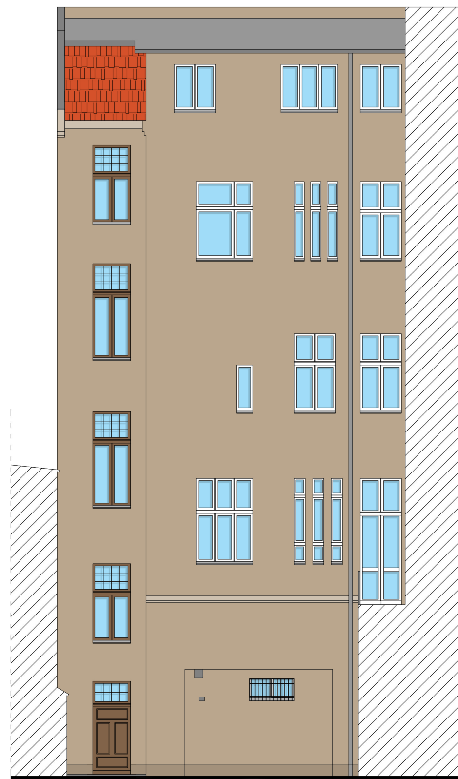
ELEWACJA PODWÓRZOWA- POŁUDNIOWA SKALA 1:100
