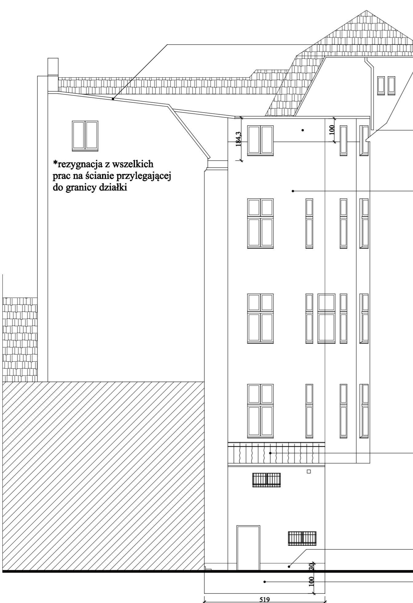
ELEWACJA PODWÓRZOWA- PÓŁNOCNA SKALA 1:100
