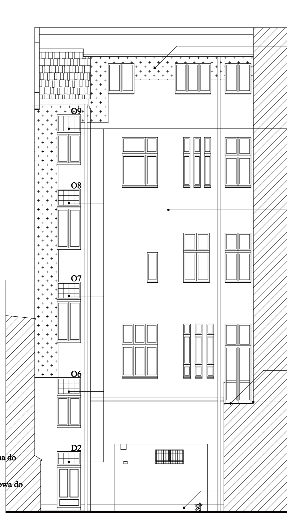
ELEWACJA PODWÓRZOWA- POŁUDNIOWA SKALA 1:100
