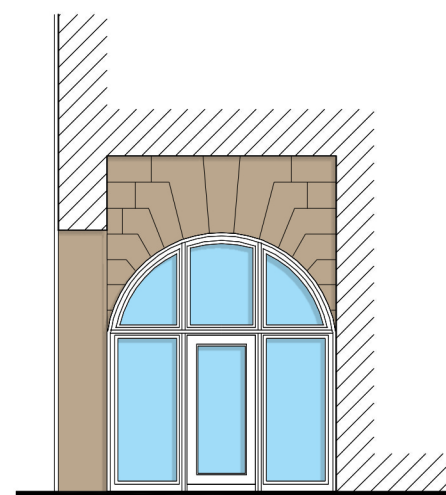
ELEWACJA ARKAD- WSCHODNIA SKALA 1:100
