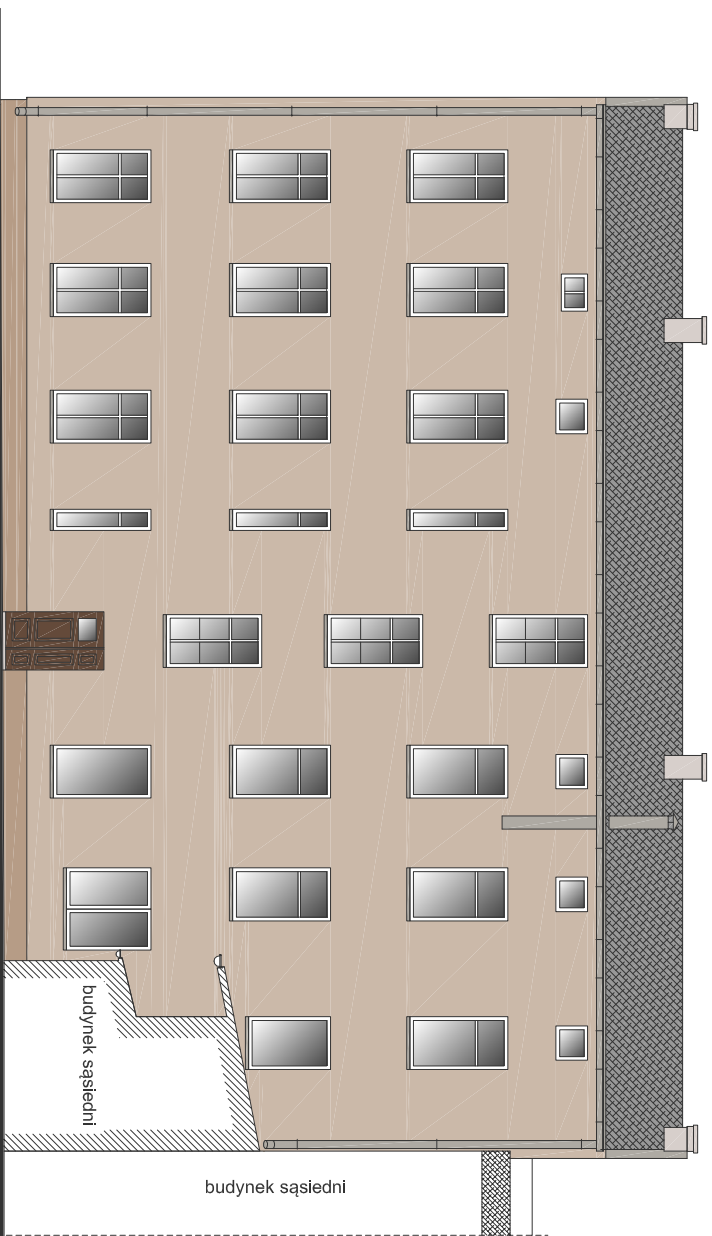
ELEWACJA POŁUDNIOWA
