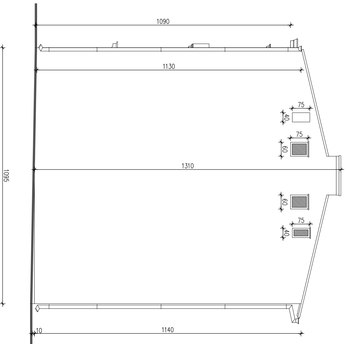
ELEWACJA ZACHODNIA
