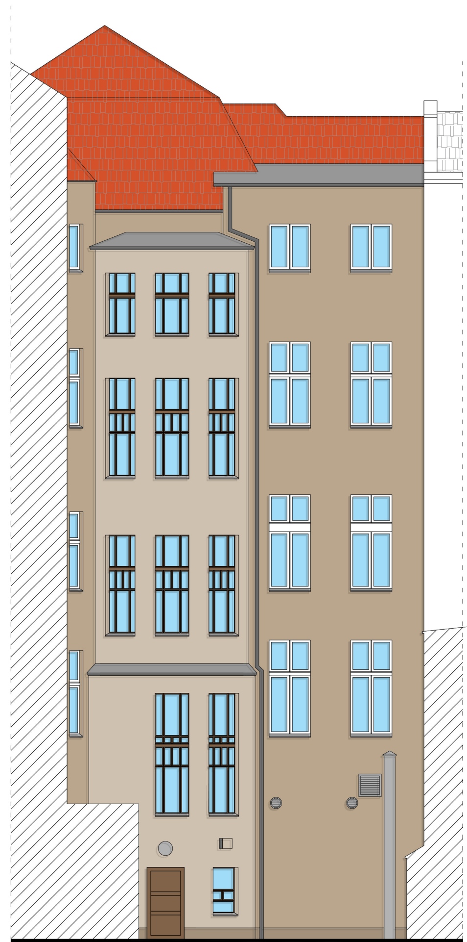
ELEWACJA PODWÓRZOWA- ZACHODNIA SKALA 1:100
