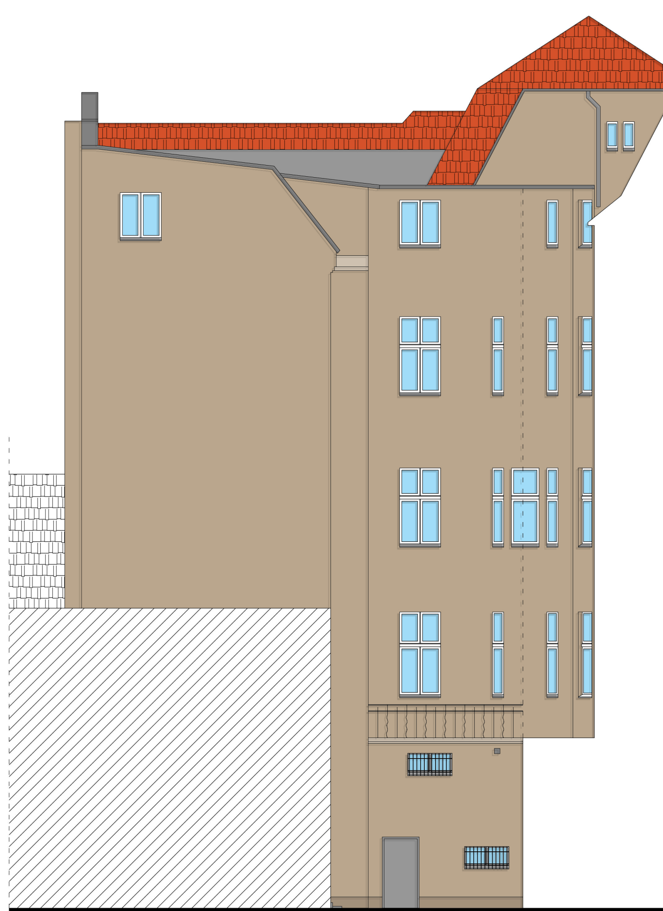
ELEWACJA PODWÓRZOWA- PÓŁNOCNA SKALA 1:100
