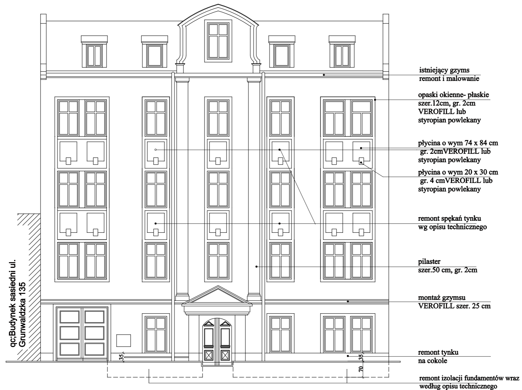
ELEWACJA FRONTOWA PÓŁNOCNO- WSCHODNIA 1:100
