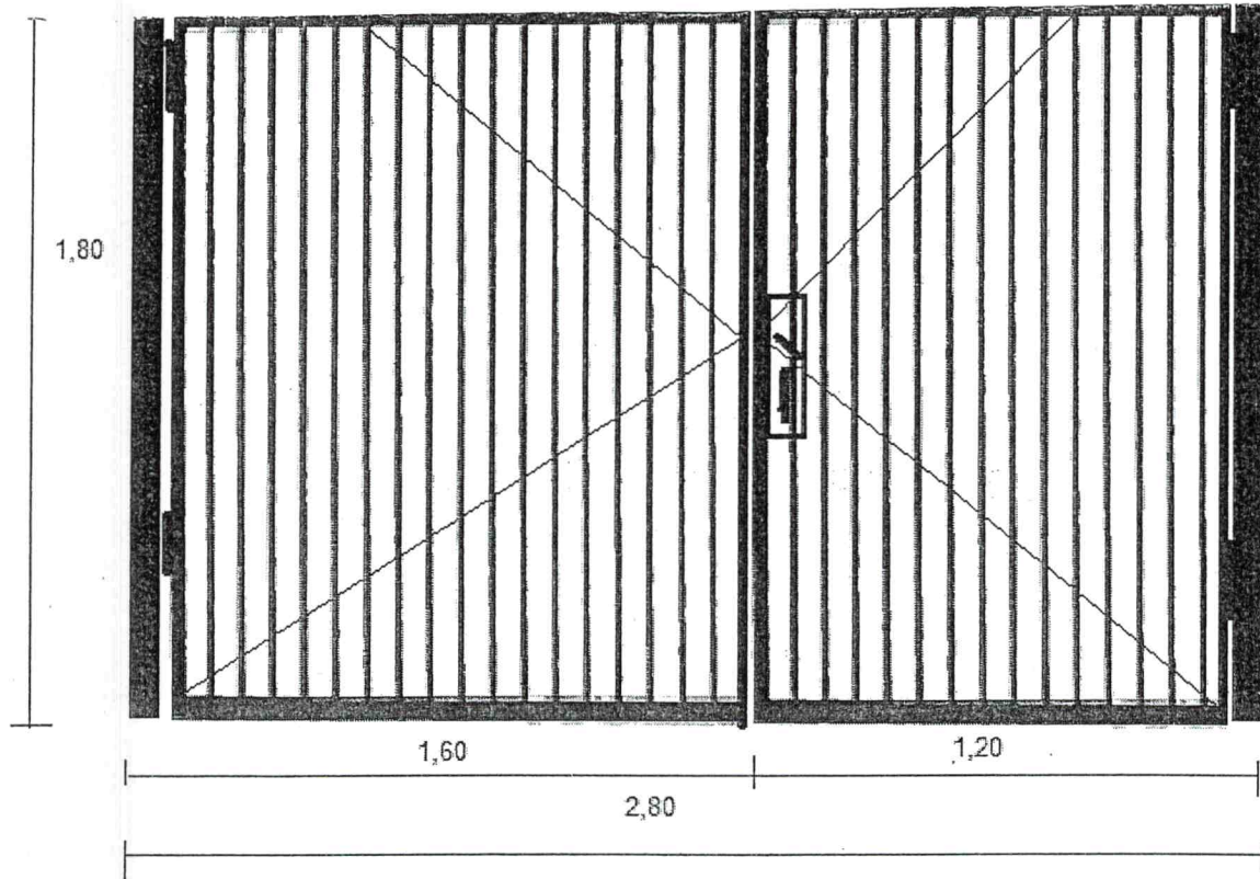
Brama stalowa z profili zamkniętych usytuowana we wjeździe budynku
