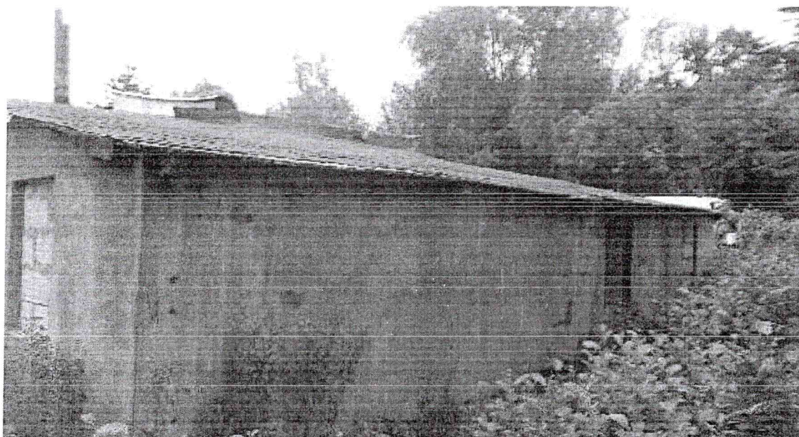
fot. nr 1 Widok ogólny budynku przewidzianego do rozbiórki – część wysoka. Widoczne ugięcia więźby dachowej oraz zamurowane otwory okienne.
