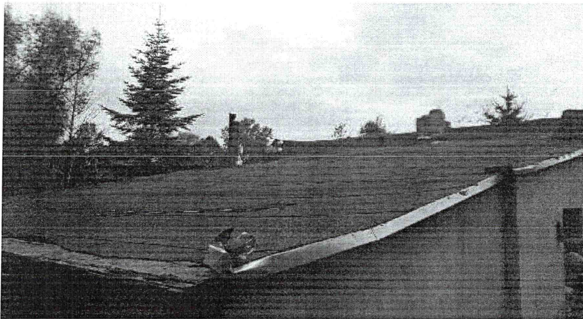
fot. nr 4 poszycie dachu – ubytki papy oraz usunięte i uszkodzone obróbki blacharskie.
