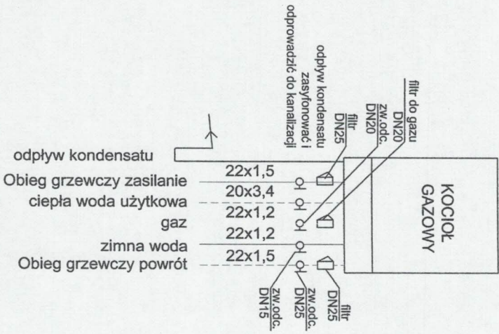
Szczegóły podłączenia kotła do instalacji gazu, c.o. i c.w.u.
