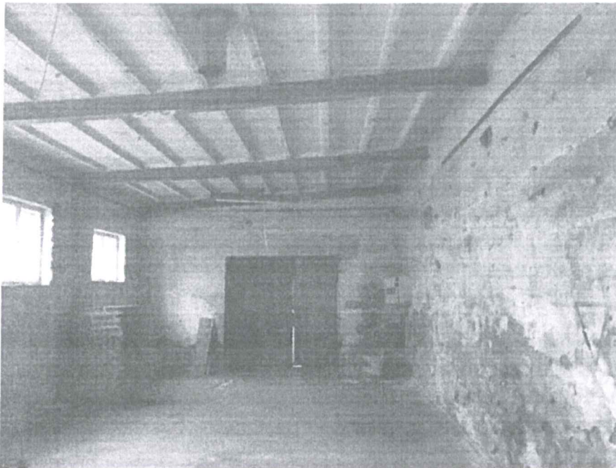
fot. nr 5 Wnętrze budynku nr 78:1 – konstrukcja dachu betonowe płyty prefabrykowane oparte na dźwigarach stalowych, posadzka przemysłowa betonowa, ściany murowane.
